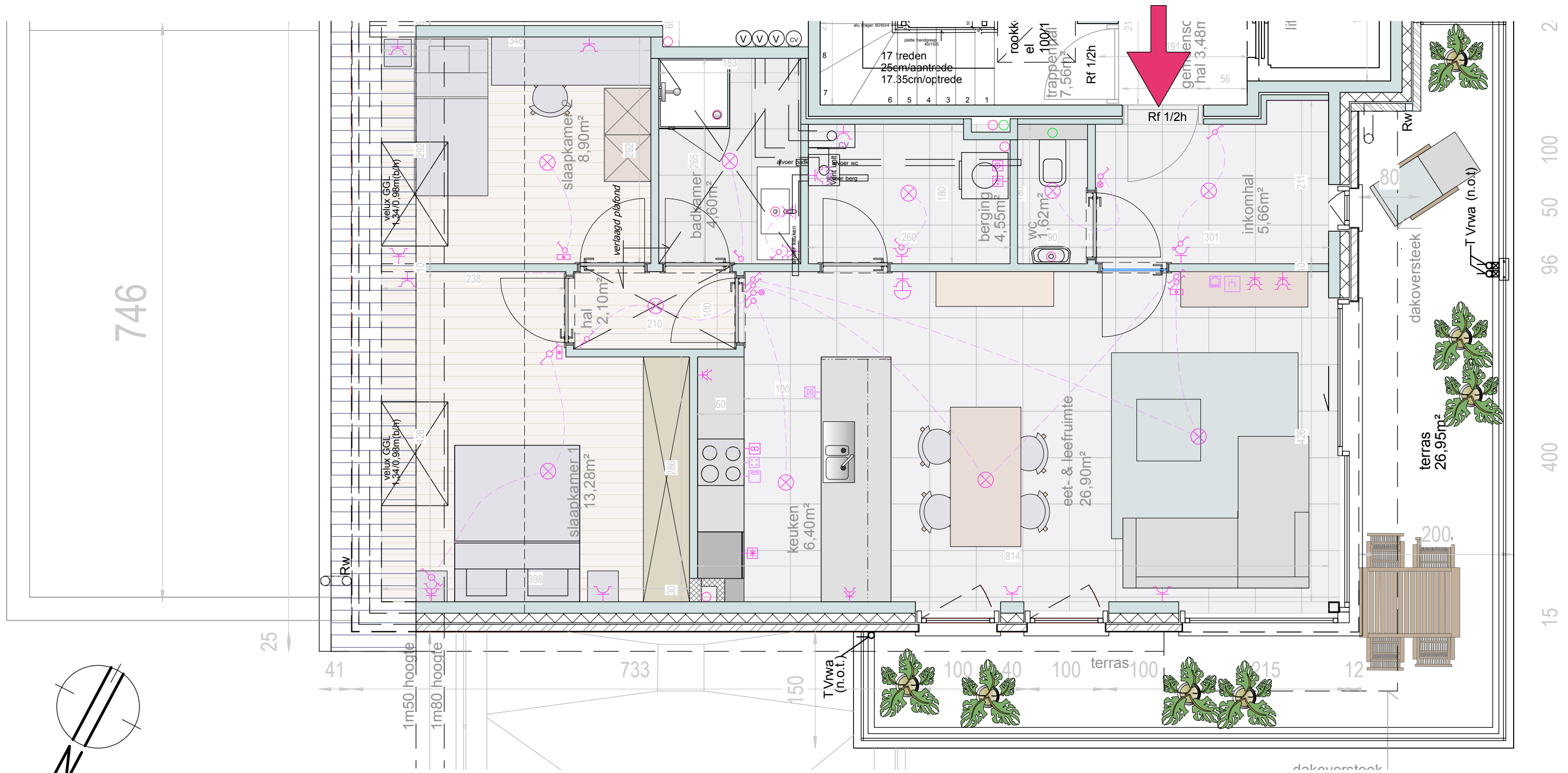
TWEEDE VERDIEPING N+2
